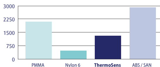
Модул на огъване (MPa)
