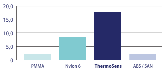
Якост на удар по Шарпи (kJ/m 2 )
